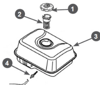
Рис. 19 Обслуживание топливных фильтров
