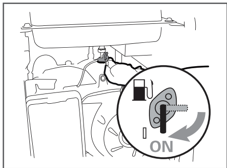
Рис. 11 Открытие топливного крана
