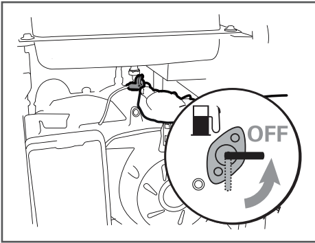
Рис. 18 Закрытие топливного крана
