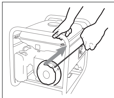
Рис. 14 Запуск двигателя ручным стартером
